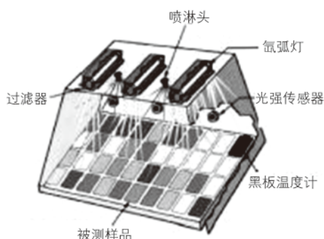
图3 平板氙灯试验箱示意图
