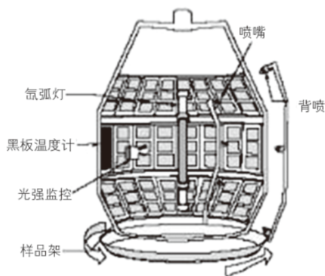
图4 旋转氙灯试验箱示意图
